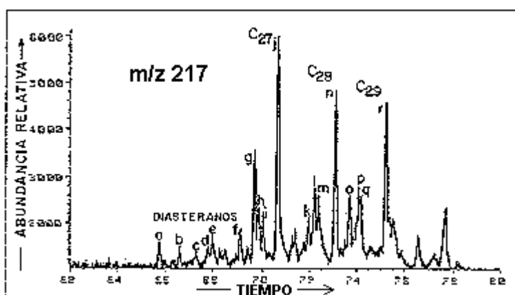
Distribución de biomarcadores esteranos m/z 217 de la impregnación de petróleo Imp-2 (Tomado de: Del Olio, 1993)
