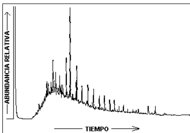
Cromatograma de la fracción saturada de la impregnación de petróleo Imp-2 (Tomado de: Del Olio, 1993)
