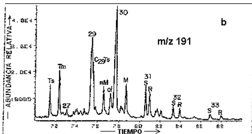
Comparación de distribución de terpanos de (a) Abundancia y (b) Imp-2 (Tomado de: Del Olio, 1993)
