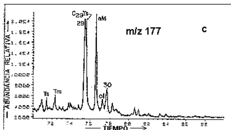
Distribución de biomarcadores terpanos (a) y hopanos m/z 191(b) y m/z 177(c) de la impregnación de petróleo Imp-2
