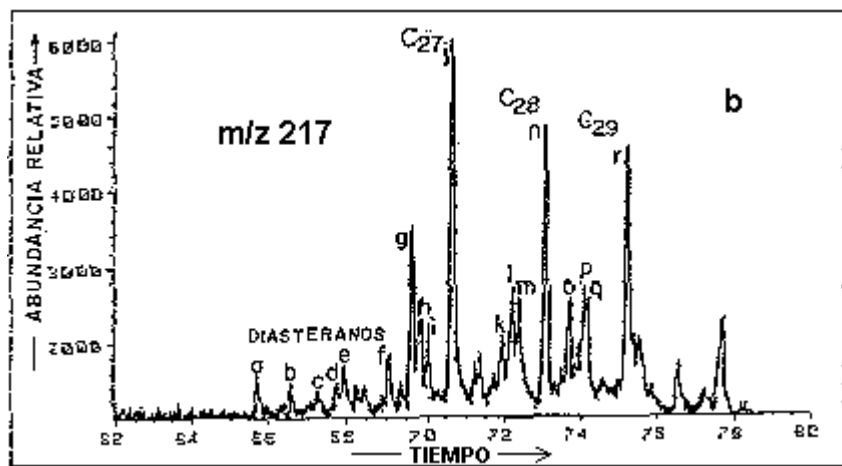
Comparación de distribución de esteranos de (a) Abundancia y (b) Imp-2 (Tomado de: Del Olio, 1993)
