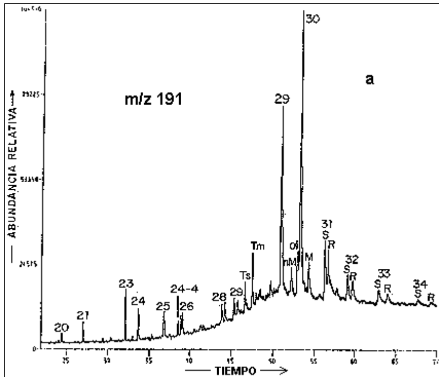
Comparación de distribución de esteranos de (a) Abundancia y (b) Imp-2 (Tomado de: Del Olio, 1993)
